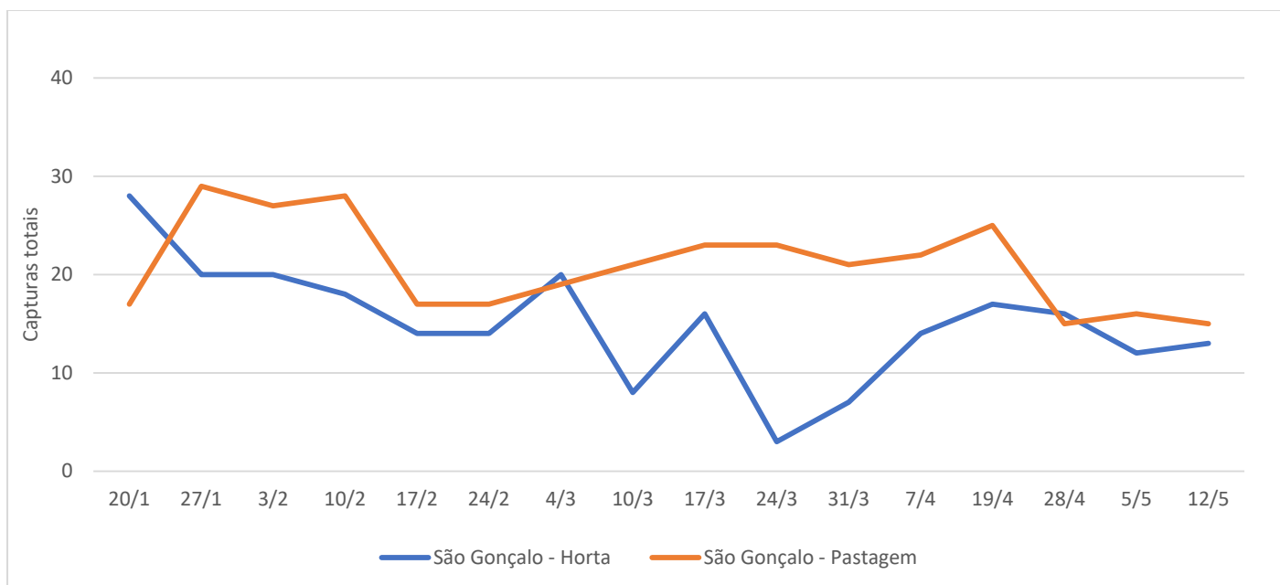
Figura 1 e 1ª - Evolução das capturas de adultos de S. littoralis por armadilha e por dia, nas parcelas monitorizadas nas freguesias de Capelas, Água de Pau e Furnas (acima) e São Gonçalo (abaixo) da ilha de S. Miguel, no ano de 2022.
